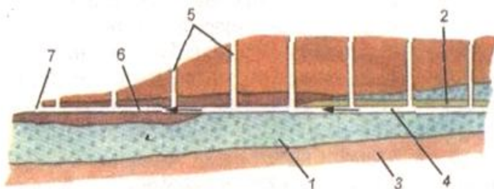
–расм. коризларнинг конструктив ечими ва қирқими: 1–сувли қатлам; 2 –қум; 3–лой қавати; 4–сув йиғадиган лаҳм; 5–вертикал қудуқлар 6–сув ўтказадиган лаҳм; 7–сув олиб чиқадиган канал.
