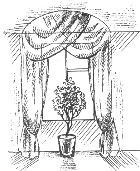
Рис. 9.а Солитер
