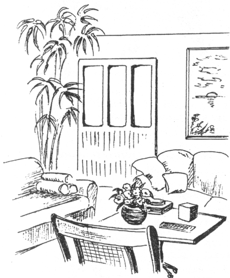
Рис. 9. Солитер
