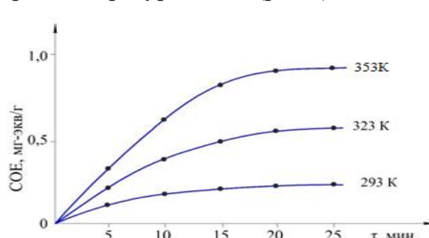
Рис.4. Кинетика окисления омыленного нитрона гипохлоридом натрия (NaClO)
