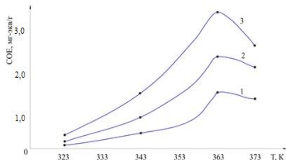
1, 2, 3-соответственно 6 г/л; 9 г/л; 12 г/л; Рис. 6. Изменение СОЕ модифицированного нитрона в зависимости от температуры реакции при концентрациях гидросиламина
