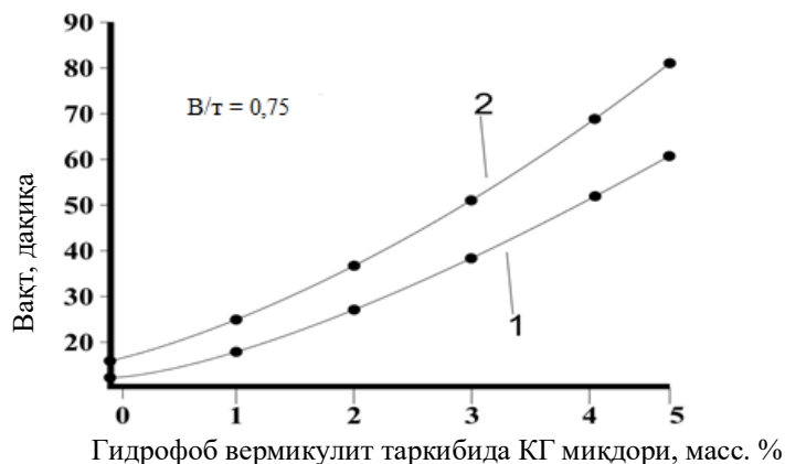
7-расм. Кўпчитилган вермикулитнинг гидрофобланиш даражасининг гипс-вермикулитли сувоқ аралашмасининг қотиш даврига таъсири: 1–қотиш даврининг бошланиши; 2–қотиш даврининг тугаши
