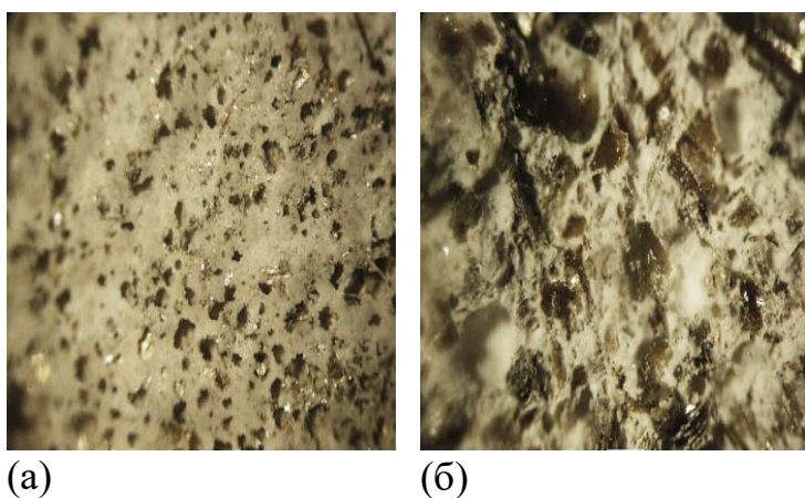
6-расм. Гипс-вермикулитли сувоқ аралашмасининг етти кунда қотишидан сўнг кўндаланг синиш сирт юзаси рельефи
