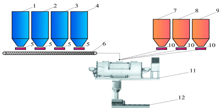
Рис. 9. Технологическая схема производства гипсо-вермикулитовых теплоизоляционных смесей:
