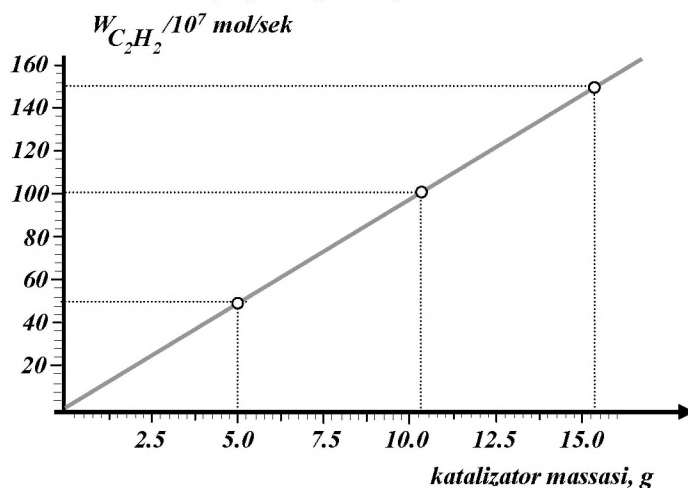
1-расм. Ацетилен сарфининг катализатор миқдорига боғлиқлиги (синтез шароити: t = 300^\circ\text{C} ; P_{C_2H_2} = 0.1 \text{ атм} ). Катализатор №25
