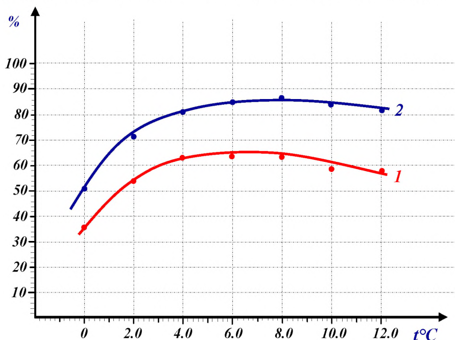
Рис. 2. Температурная зависимость реакции азосоединения пирролдиазоуксусной кислоты с этиловым эфиром: 1) время воздействия -6 часов; 2) время воздействия- 10 часов;
