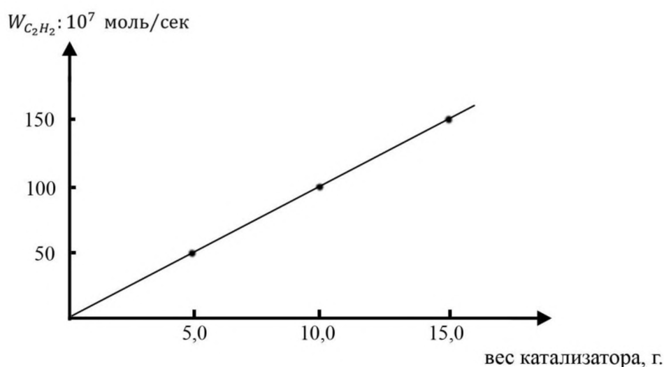
Рис. 1. Зависимость расхода ацетилена от количества катализатора (условия синтеза: t = 300^\circ\text{C} ; P_{C_2H_2} = 0.1 атм). Катализатор №25
