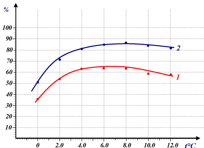
2-расм. Пиррол диазосирка кислота этил эфири азокўшиш реакциясига хароратнинг боғлиқлиги: 1- таъсир вақти 6 соат; 2-таъсир вақти 10 соат
