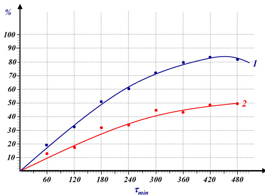
Рис.5 .Зависимость природы катализатора от реакций азосоединения:
