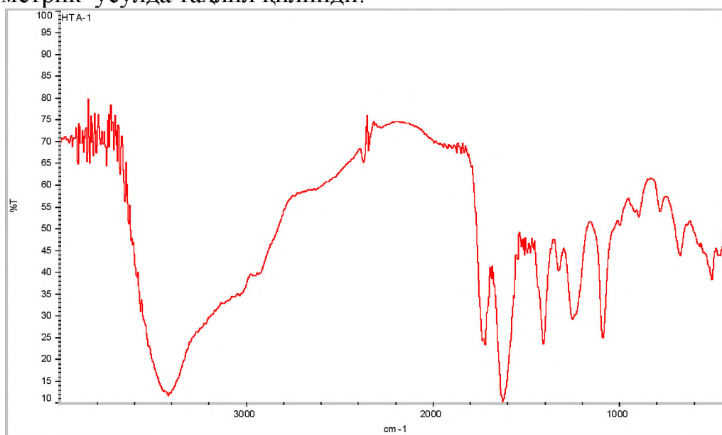
3-расм. \alpha -Карбоксиметилпирролнинг ИҚ-спектри
