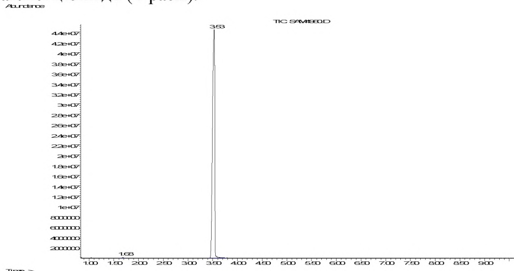
4-расм. \alpha -Карбоксиметилпирролнинг хромато-масс спектри
