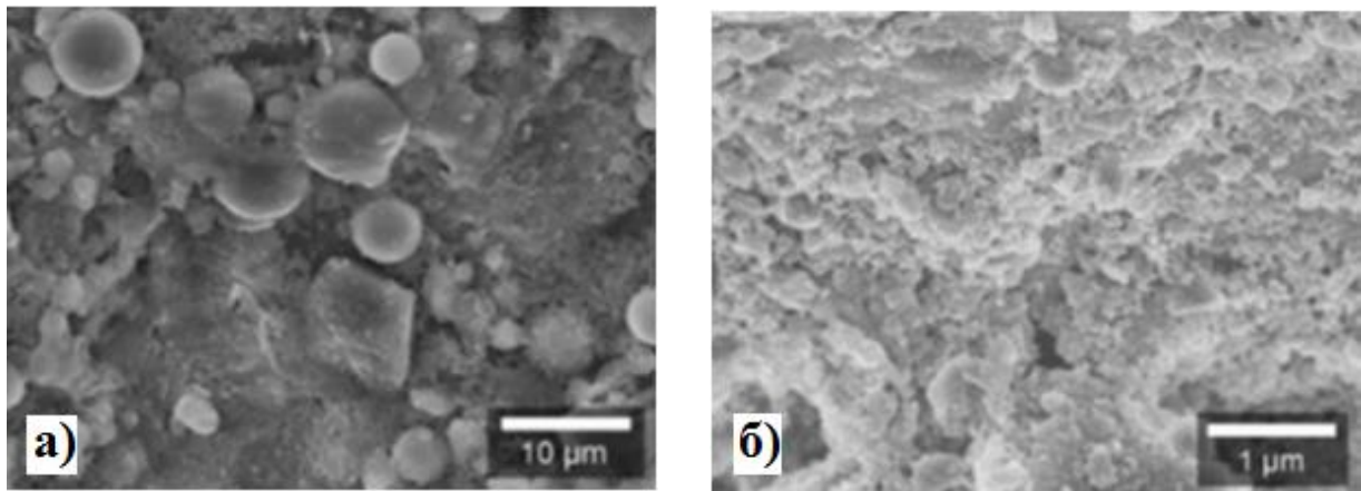
5-расм. Олтингугуртли бетоннинг СЭМ тасвири.
