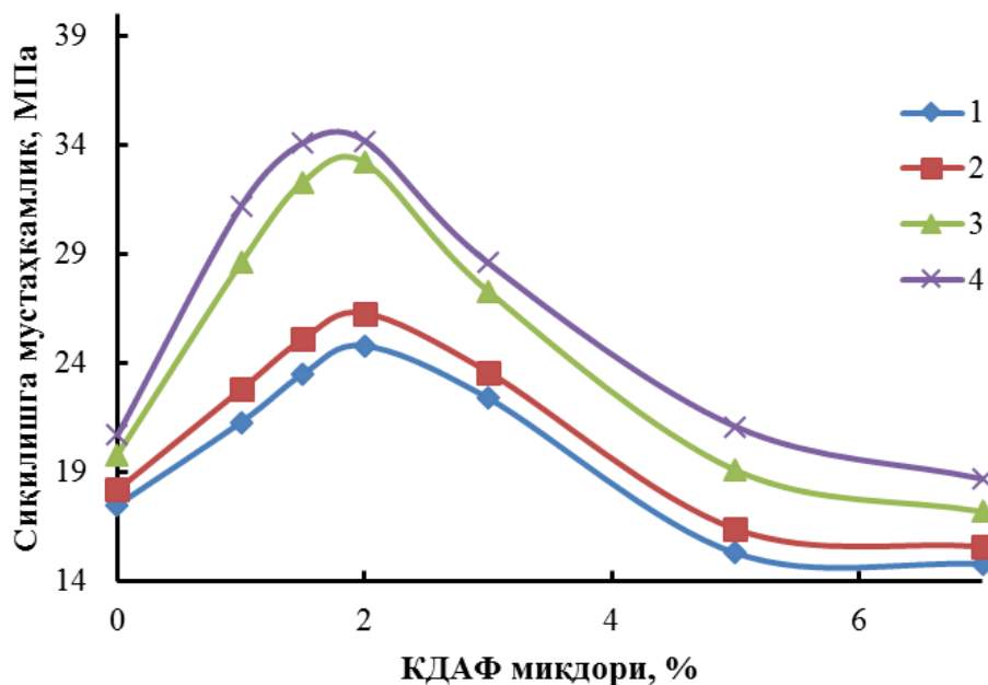
6-расм. Олтингугурт-кул асосидаги композициялар сиқилишга мустаҳкамлигининг модификацияловчи КДАМ миқдorigа боғлиқлиги: тебранма зичлаш (1, 2) ва сиқиш (3, 4) усулида 1, 3- 30 минут; 2, 4-60 минут давомида олинган намуналар
