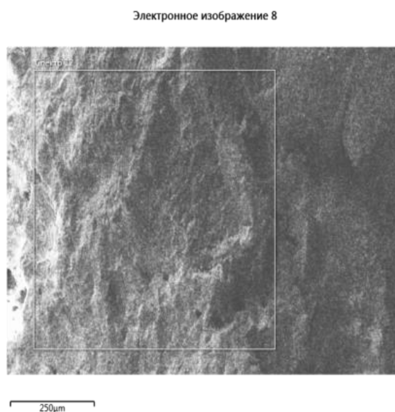
Рис. 3. СЭМ анализы серного бетона.
