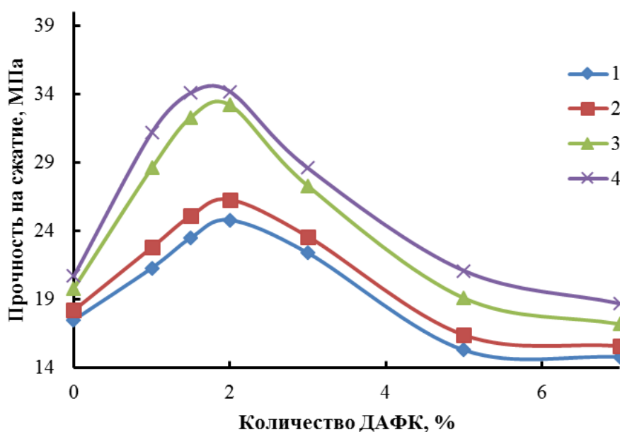
Рис.6 . Прочность на сжатие сернозолоуносных композиций: виброуплотнение (1, 2) и сжатие (3, 4), с различным содержанием модифицирующей добавки ДАФК и временем синтеза: 1, 3- 30 минут; 2, 4-60
