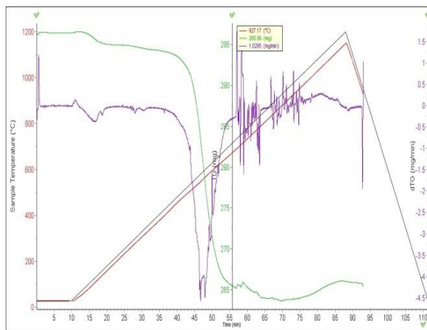
Рис. 2. ДТГ и ТГ анализ серобетона.
