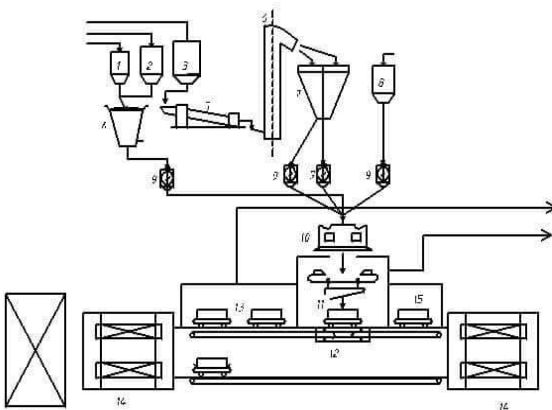
7-расм. Олтингурутли бетон олишнинг технологик схемаси:
