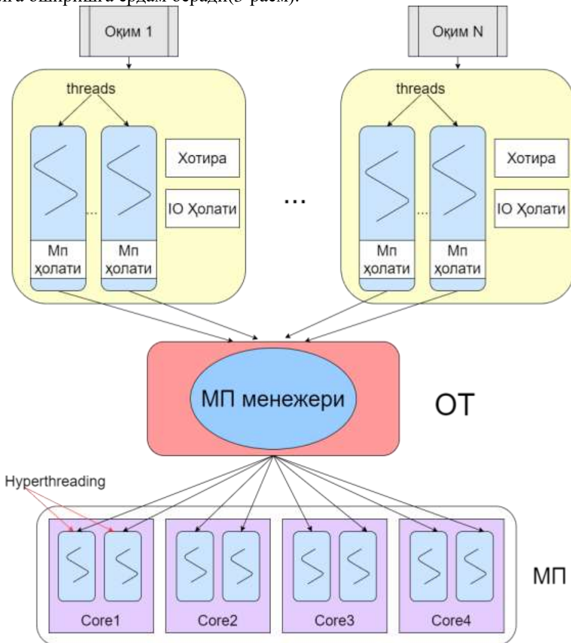
3-расм. Hyper-Threading технологиясидан фойдаланиб процессордаги оқимларини тавсифлаш.
