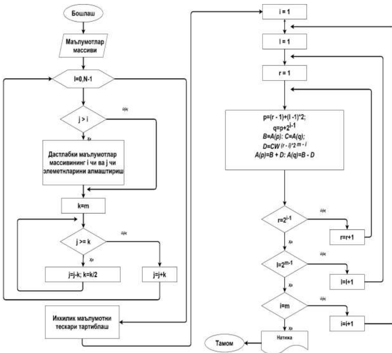
4-расм. Маълумотлар массивига паралелл ишлов бериш алгоритмининг блок-схемаси.
