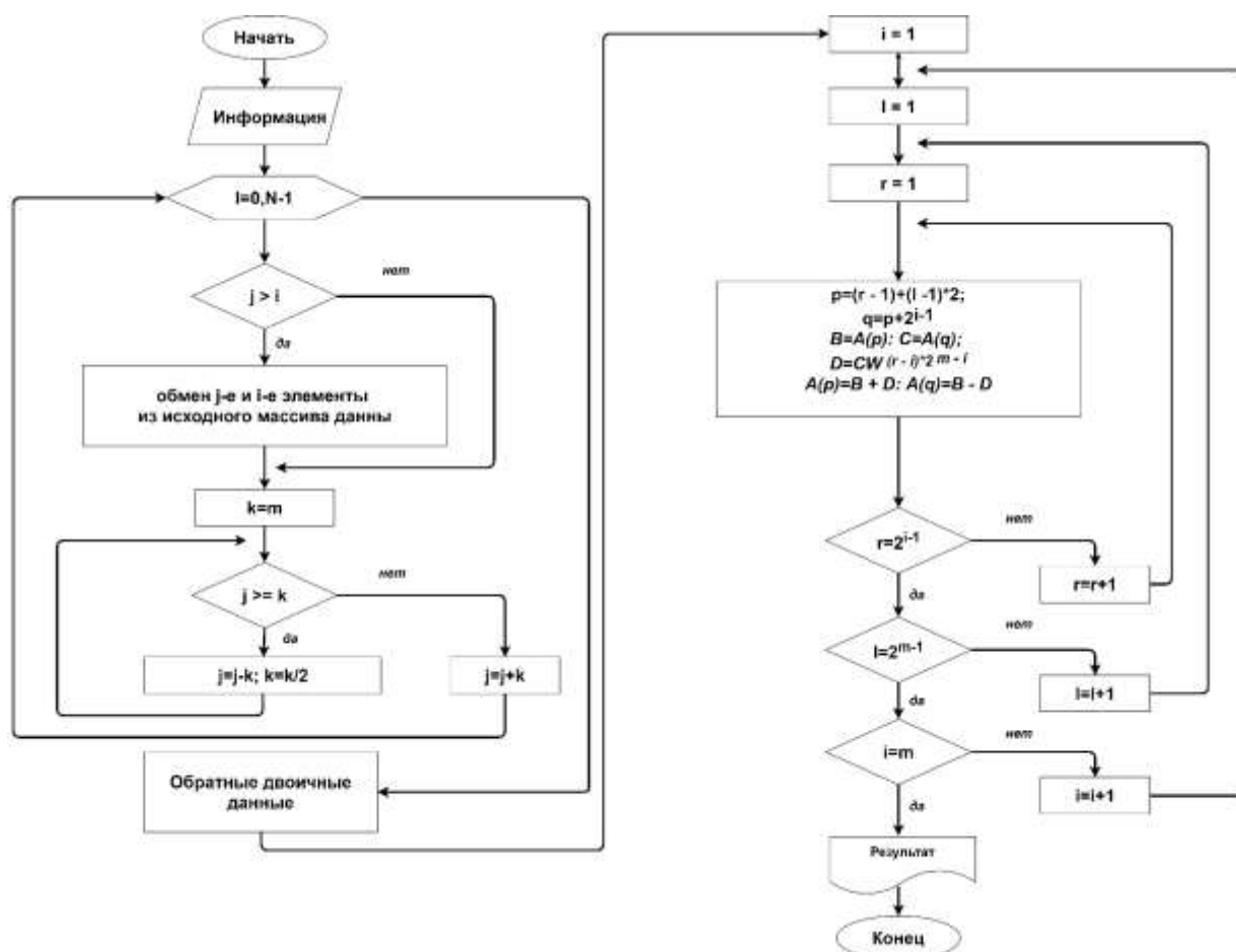
Рис. 4. Блок-схема алгоритма параллельной обработки массивов данных
