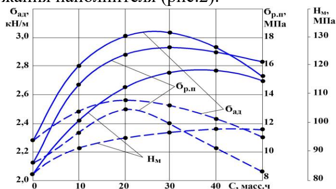
Рис.2. Зависимость свойств модифицированных ультразвуком (-) и немодифицированных (- -) композиционных фурано-эпоксидных покрытий от содержания чешуйчатого графита.
