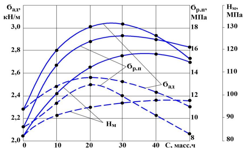
2-расм. Ультратовуш билан модификацияланган (-) ва модификацияланмаган (---) композицион фуран-эпоксид қопламаларнинг графит миқдorigа боғлиқлиги
