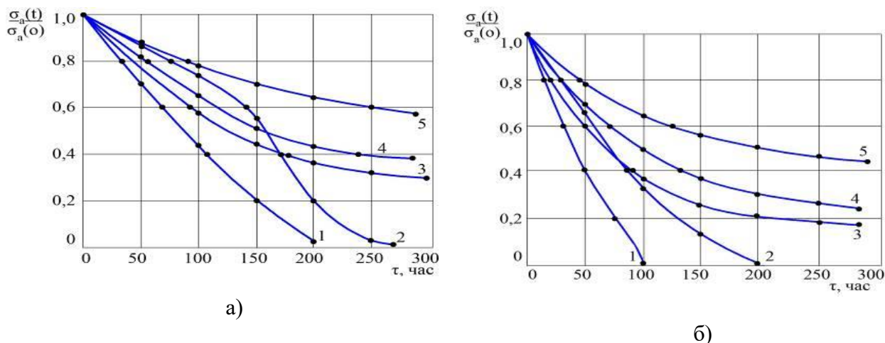
Рис. 3. Изменение адгезионной прочности фурано-эпоксидных полимерных покрытий необработанных и обработанных ультразвуком к стальной подложке в различных агрессивных средах
