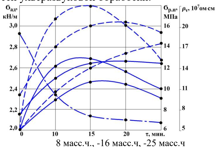
Рис.1. Зависимость адгезионной прочности, прочности при растяжении и удельного объемного сопротивления композиционных фурано-эпоксидных покрытий от продолжительности воздействия ультразвука при развличных содержаниях алюминиевой пудры
