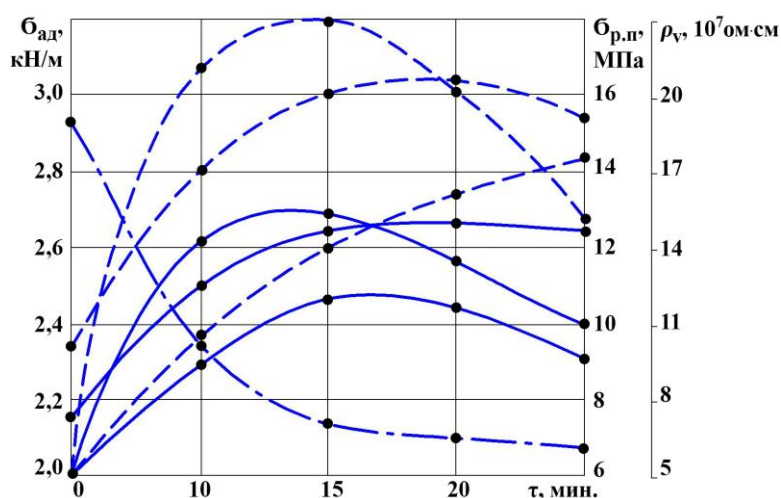
1-расм. Композицион фуран-эпоксид қопламаларининг адгезион мустаҳкамлик, тортишиш кучи ва солиштирма ҳажм қаршилиги ултратовуш давомийилигига таъсири алюминий кукунининг хар хил таркибига боғлиқлиги
