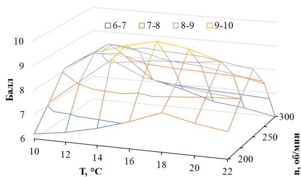
Рис. 10. Влияние температуры и скорости вращения вала на органолептические и реологические свойства маргарина при охлаждении эмульсии.
