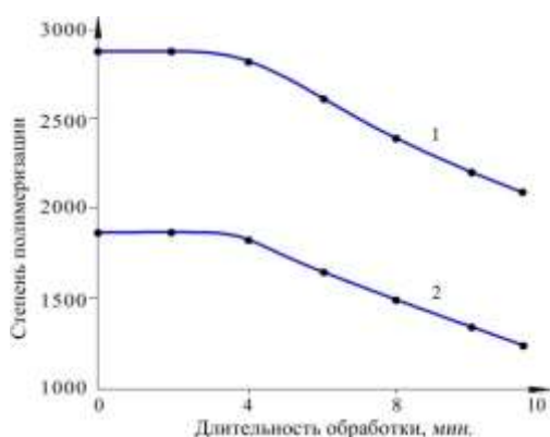
Рис. 4. Изменение степени полимеризации волокон в различных условиях
