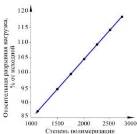
Рис. 6. Корреляционная зависимость разрывной нагрузки и степени полимеризации
