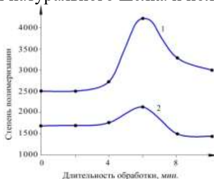
Рис. 5. Изменение степени полимеризации волокон в различных условиях
