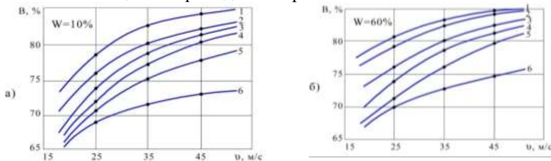
2 (а, б)-Расм. Конденцион ғўза пояси пайраҳалари миқдорининг кесиш тезлигига боғлиқлиги
