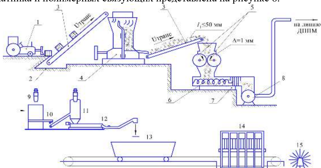
Рис. 6. Схема технологической линии производства древесно-пластиковых плитных материалов из стеблей хлопчатника и полимерных связующих
