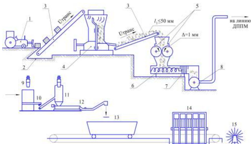
6-Расм. Ғўза пояси ва полимер боғловчилар асосида ёғоч пластик плитали материаллар ишлаб чиқариш технологик линия схемаси
