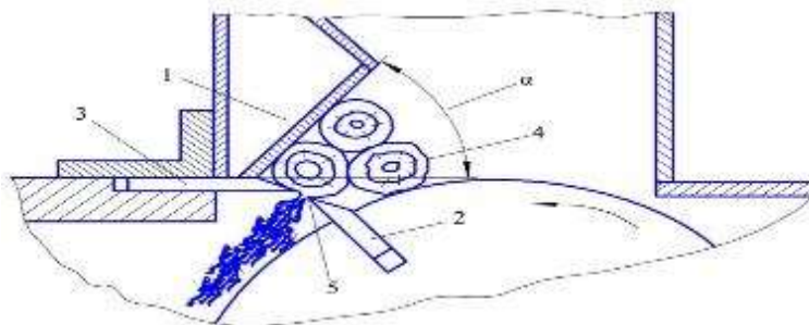
1.Накладка. 2.Нож. 3.Контрнож. 4.Щепка
