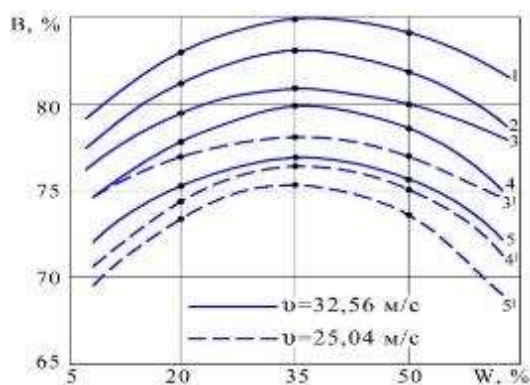
Рис. 3. Влияние влажности стеблей хлопчатника на количество конденционной щепы
