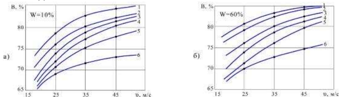
Рис. 2 (а, б) Зависимость количества конденционной щепы от скорости резания
