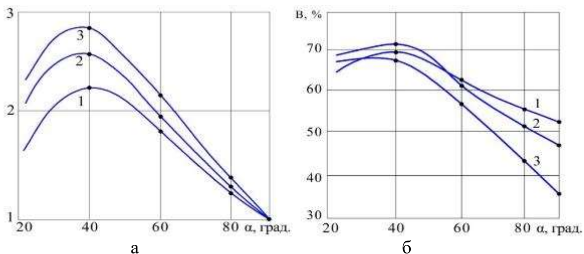
Рис. 5. Зависимость количества конденционной фракции С (а) и относительной производительности процесса измельчения К (б) от угла накладки \alpha
