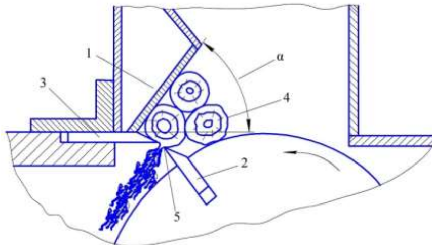
1.Қоплама. 2. Пичоқ. 3. Қарши пичоқ. 4. Пайраҳа.
