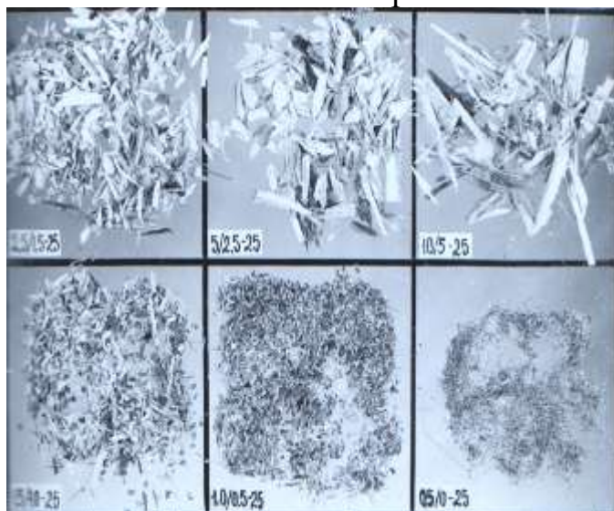
Рис. 1. Фракционный состав измельченной массы стеблей хлопчатника
