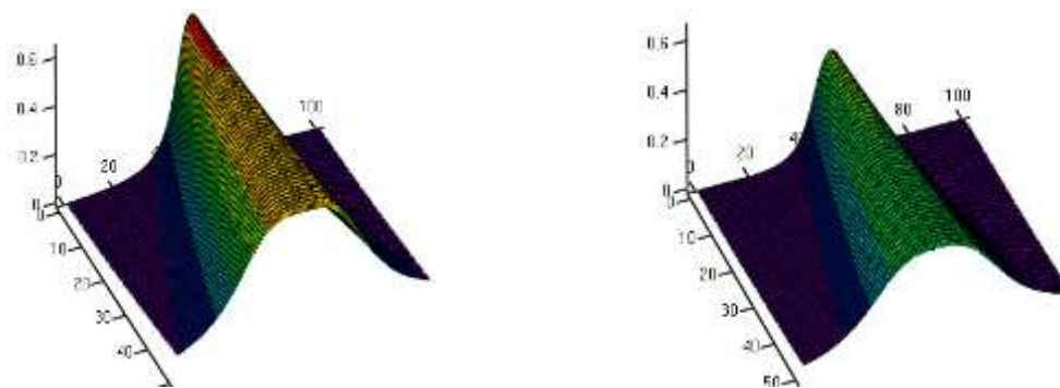
8-расм. (28)-(30) масаланинг сонли ечими. n_1=0.5, m_1=1.5, p_1=1.3 q_1=3, n_2=0.75, m_2=1.6, p_2=1.4, q_2=3.5 .
