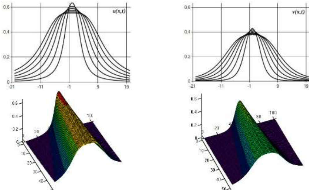
Рис 8. Численное решение задачи (28)-(30) при n1=0.5 , m1=1.5 p1=1.3 q1=3 , n2=0.75 , m2=1.6 p2=1.4 q2=3.5 .
