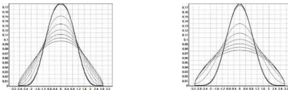
4-расм. (17)-(19) масаланинг сонли ечими. m=1.5 , p=1.75 , q=2.85 , 1) n=0 , 2) n=-0.25 .
