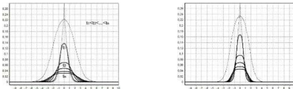
5-расм. (17)-(19) масаланинг сонли ечими m=1.5 , p=1.55 , q=2.85 , a=1.5 , 1) n=0.5 , 2) n=1 .
