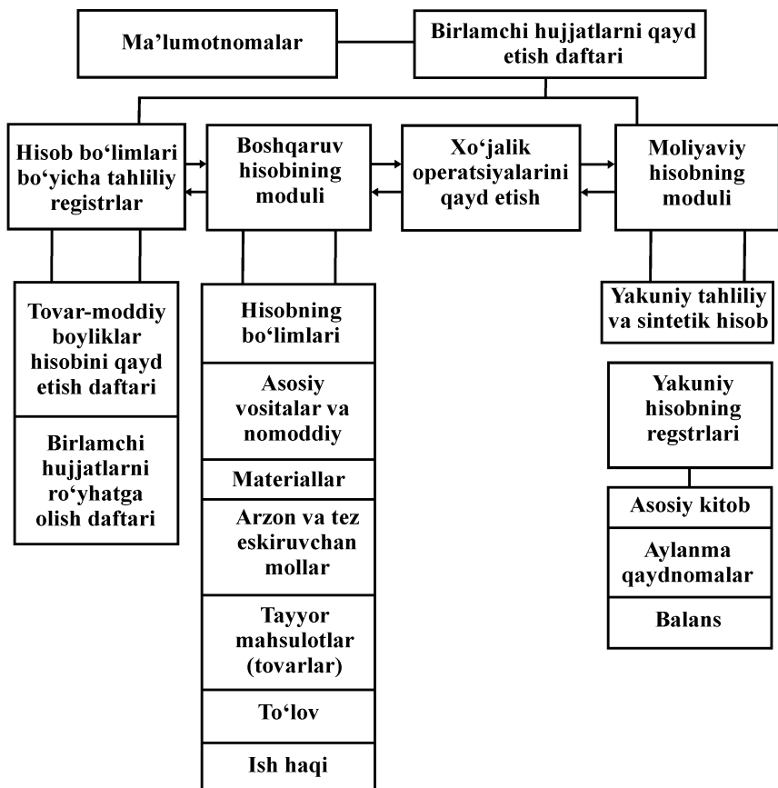
3.4-rasm. Kichik va o'rta korxonalarda buxgalteriya hisobini avtomatlashtirishning dasturiy majmuasining tarkibiy tuzilishi.
